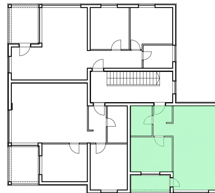
II KAT
