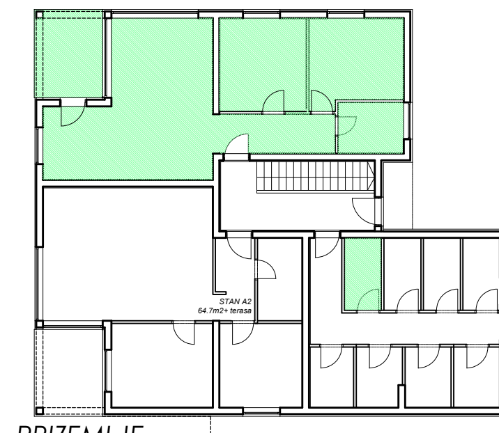
PRIZEMLJE
