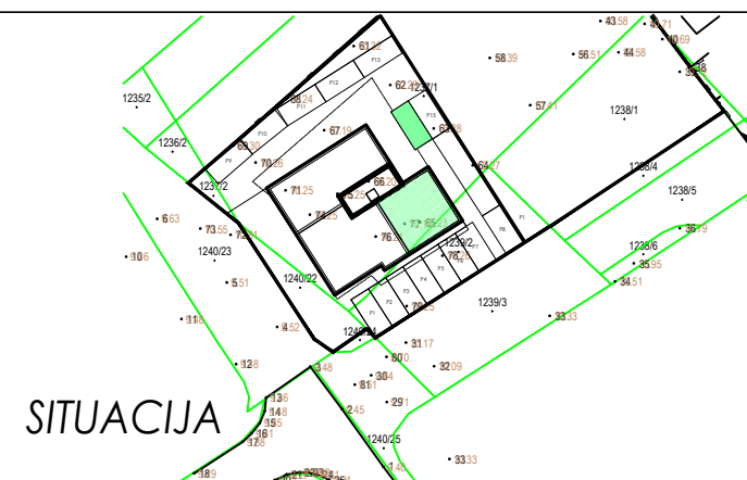
PRIZEMLJE
